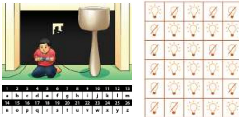
Gambar 4.33 Urutan Lampu
