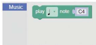
Gambar 7.9 blok [play..note..]
